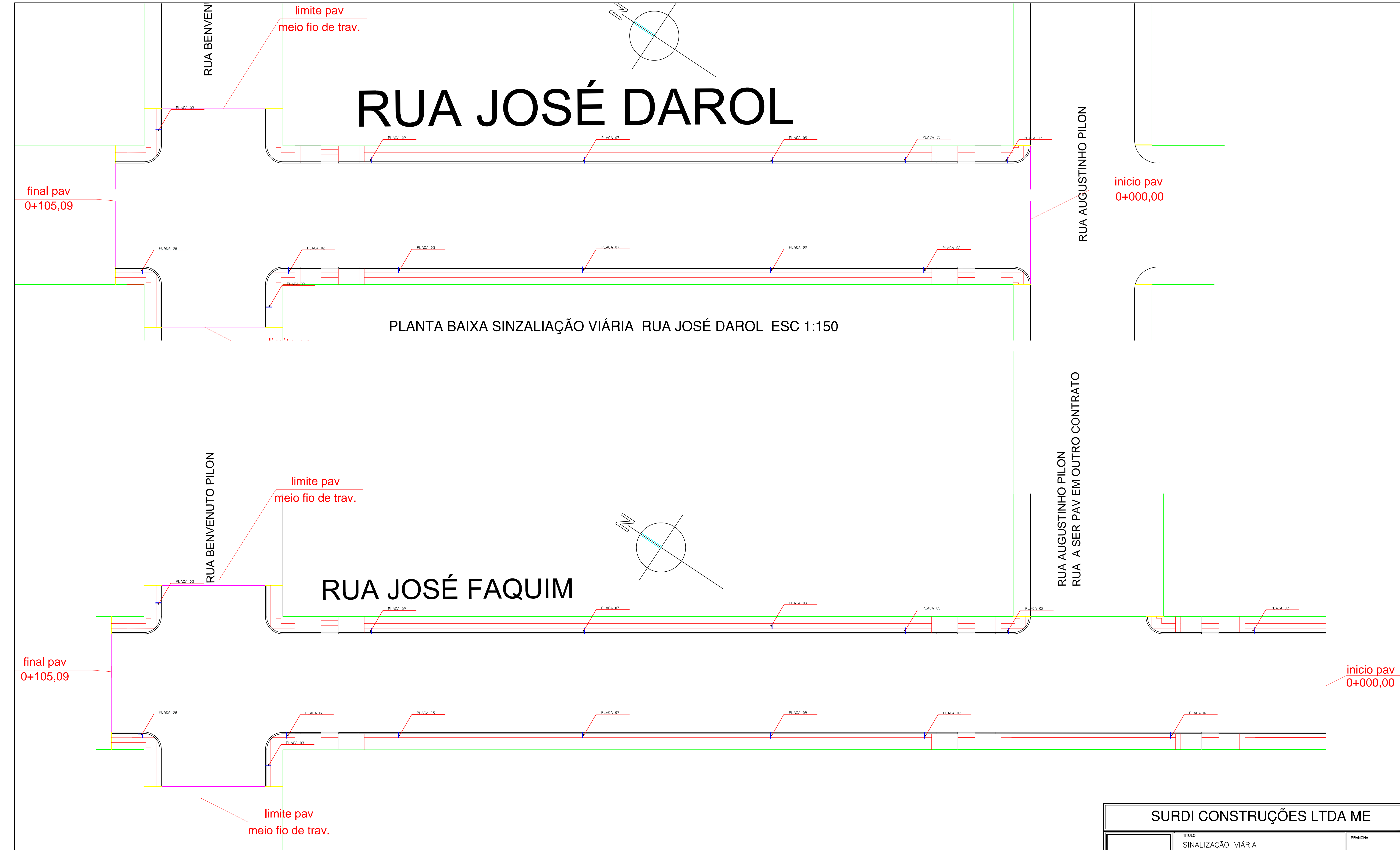
PLANTA BAIXA SINZALIAÇÃO VIÁRIA RUA JOSÉ FAQUIML ESC 1:150
