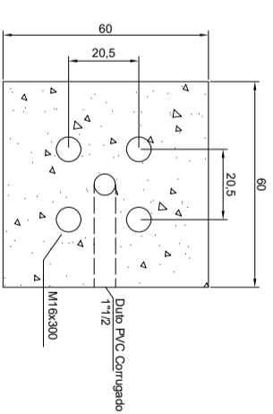
Detalhe - Vista Superior Base de Concreto p/ Postes metálicos Escala:.....Sem Nota: Cotas em cm.
