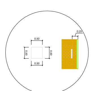
Base Balizador
